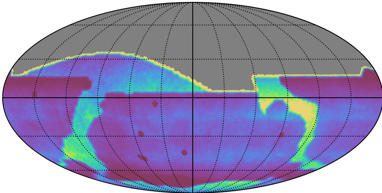
weather_cloudso35v3.5_10yrs : DCRprecision
