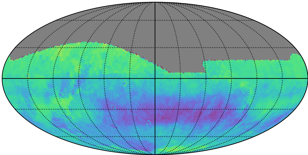
weather_cloudso35v3.5_10yrs i: Kuiper rotSkyPos
