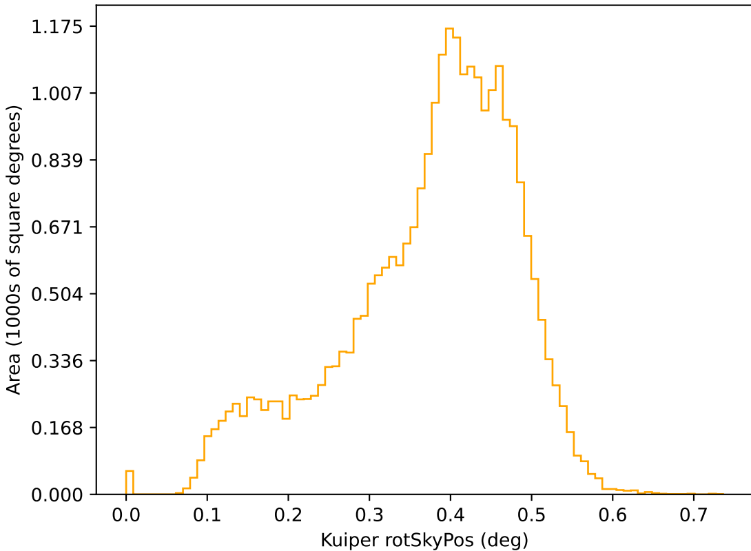
weather_cloudso35v3.5_10yrs r: Kuiper rotSkyPos
