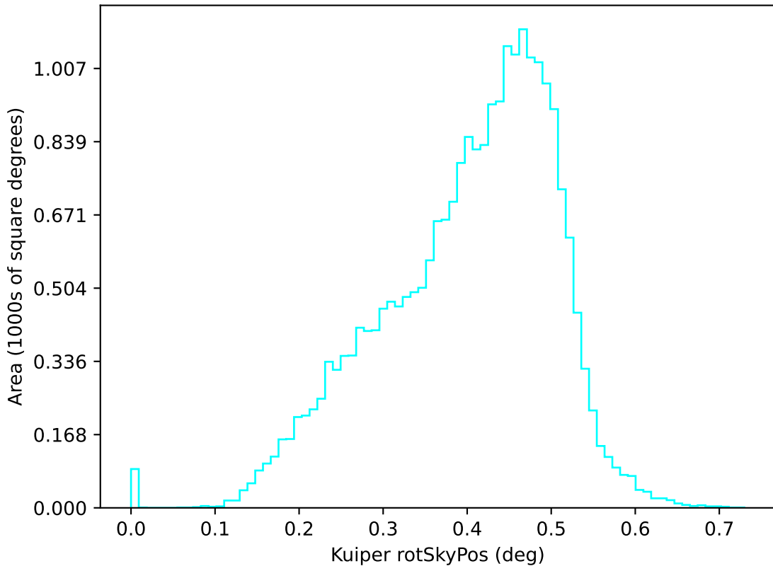
weather_cloudso35v3.5_10yrs u: Kuiper rotSkyPos
