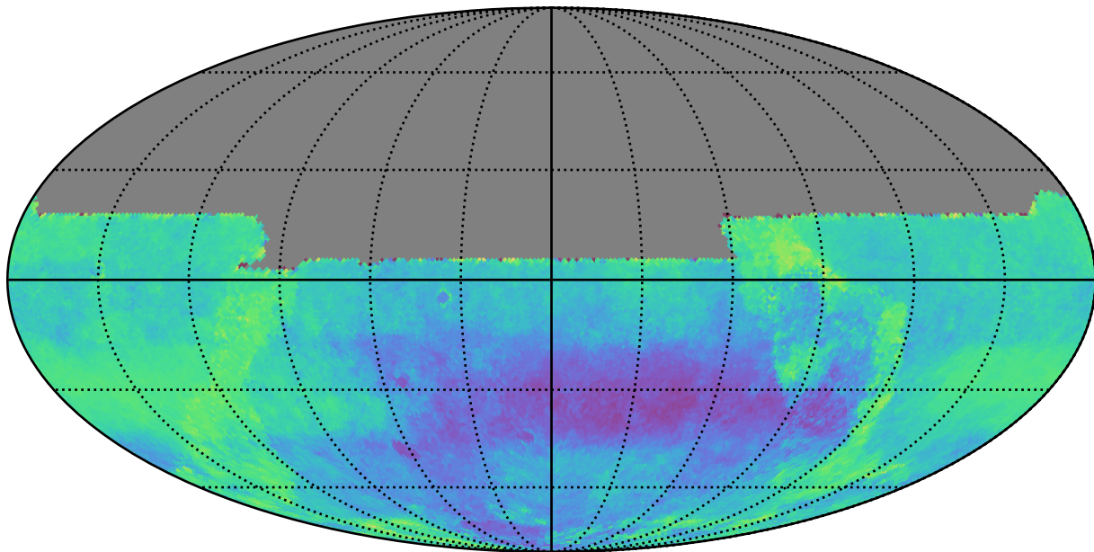
weather_cloudso35v3.5_10yrs y: Kuiper rotSkyPos
