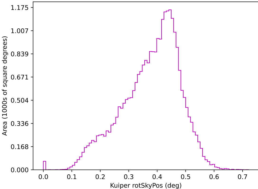
weather_cloudso35v3.5_10yrs z: Kuiper rotSkyPos
