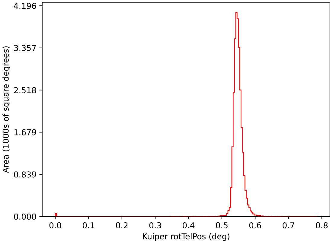
weather_cloudso35v3.5_10yrs i: Kuiper rotTelPos
