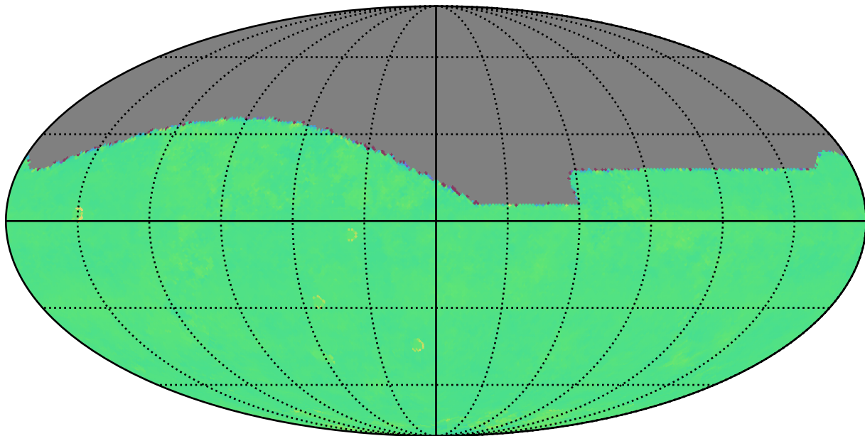
weather_cloudso35v3.5_10yrs i: Kuiper rotTelPos
