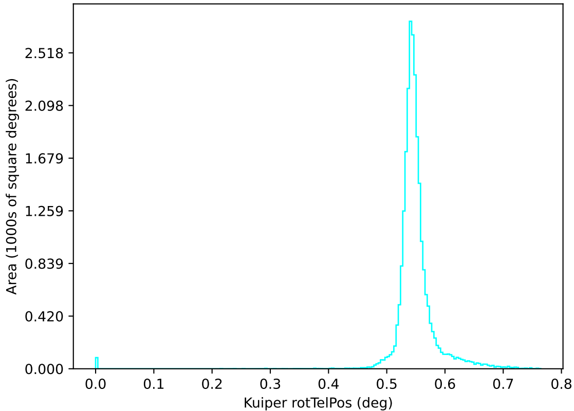
weather_cloudso35v3.5_10yrs u: Kuiper rotTelPos
