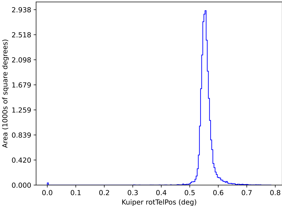
weather_cloudso35v3.5_10yrs y: Kuiper rotTelPos
