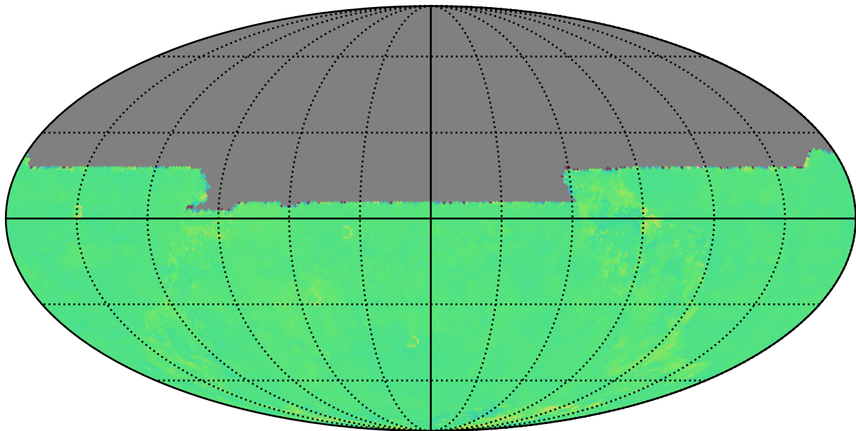
weather_cloudso35v3.5_10yrs y: Kuiper rotTelPos
