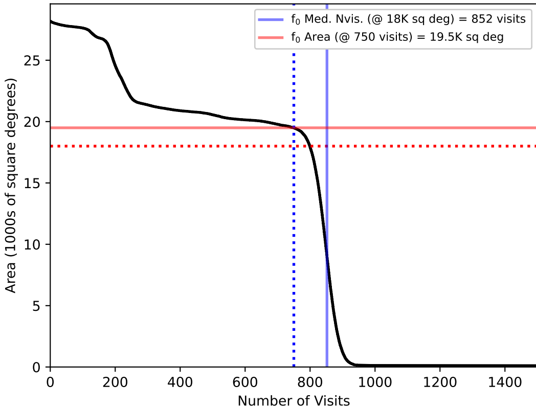
weather_cloudso35v3.5_10yrs : fO
