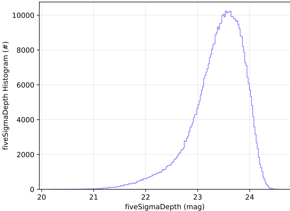
weather_cloudso35v3.5_10yrs i: fiveSigmaDepth Histogram
