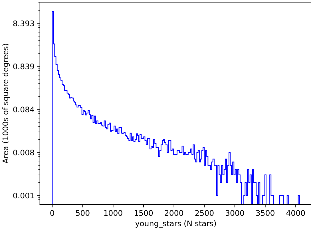
weather_cloudso35v3.5_10yrs : young_stars
