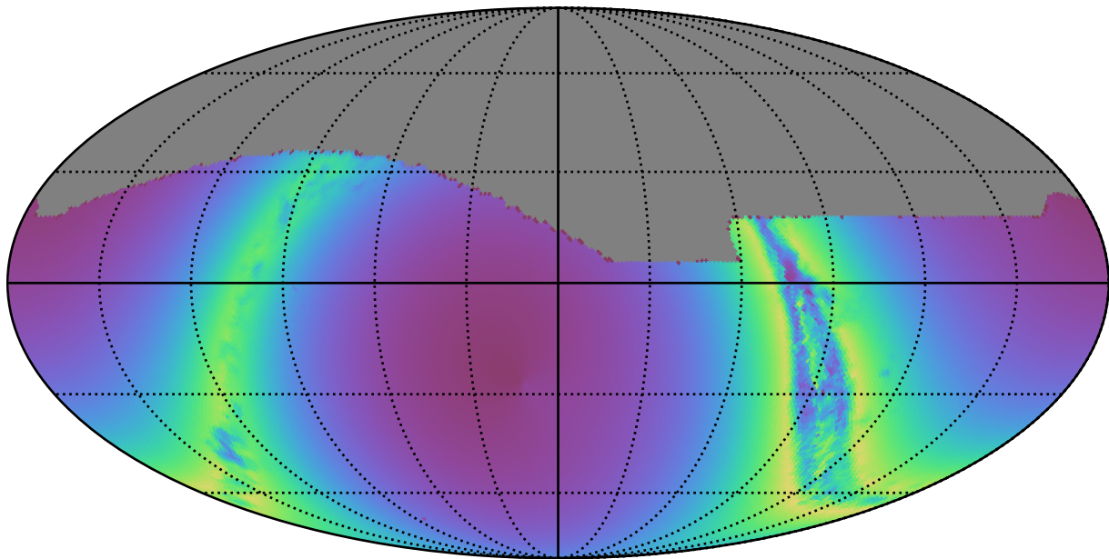
weather_cloudso35v3.5_10yrs : young_stars
