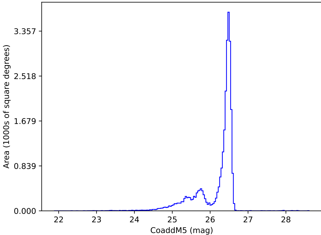
weather_cloudso36v3.5_10yrs i: CoaddM5
