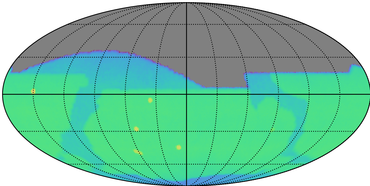
weather_cloudso36v3.5_10yrs i: CoaddM5
