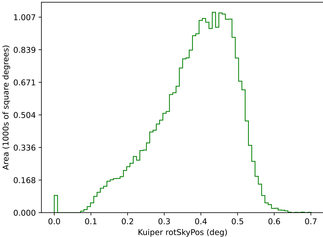
weather_cloudso36v3.5_10yrs g: Kuiper rotSkyPos
