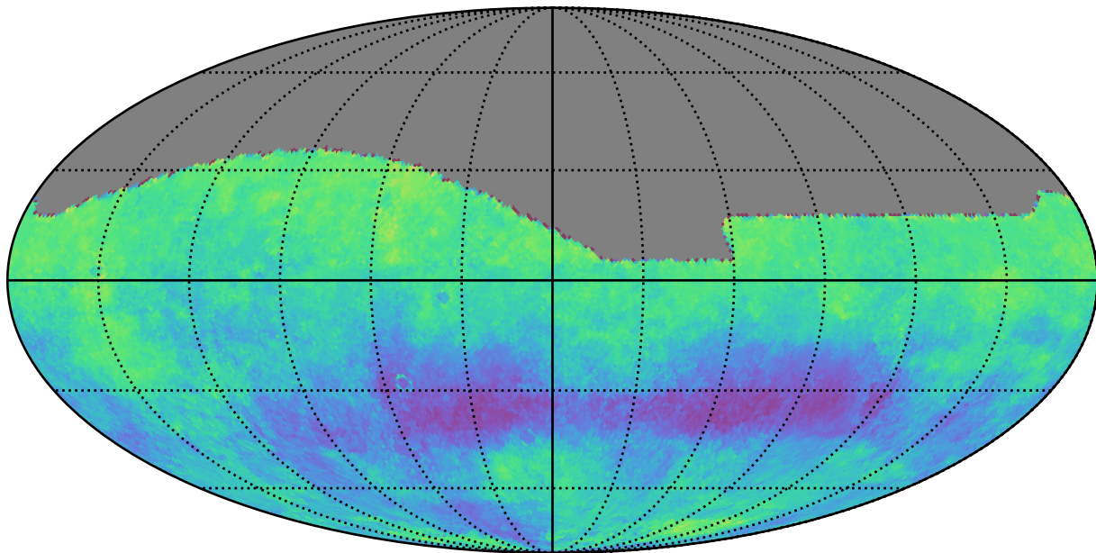
weather_cloudso36v3.5_10yrs g: Kuiper rotSkyPos
