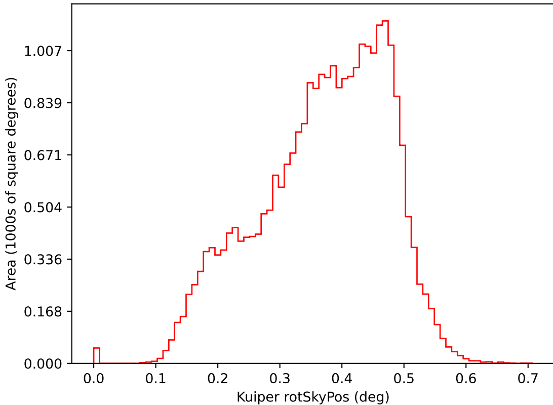
weather_cloudso36v3.5_10yrs i: Kuiper rotSkyPos
