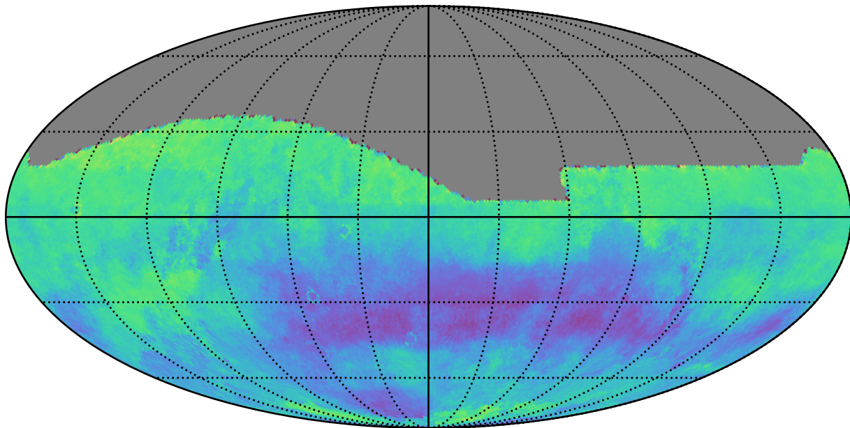
weather_cloudso36v3.5_10yrs i: Kuiper rotSkyPos
