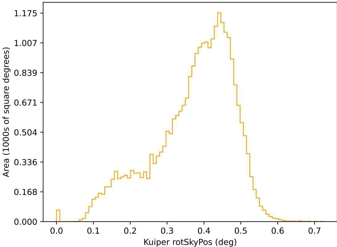
weather_cloudso36v3.5_10yrs r: Kuiper rotSkyPos
