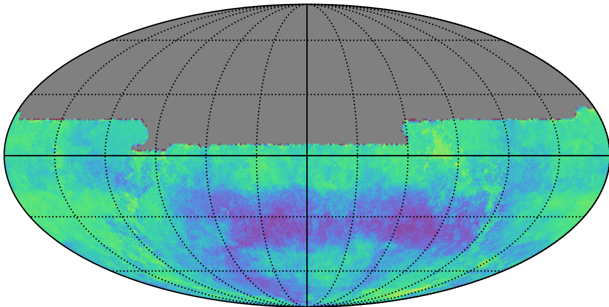
weather_cloudso36v3.5_10yrs u: Kuiper rotSkyPos
