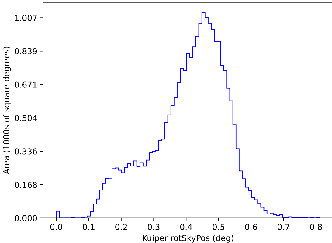
weather_cloudso36v3.5_10yrs y: Kuiper rotSkyPos
