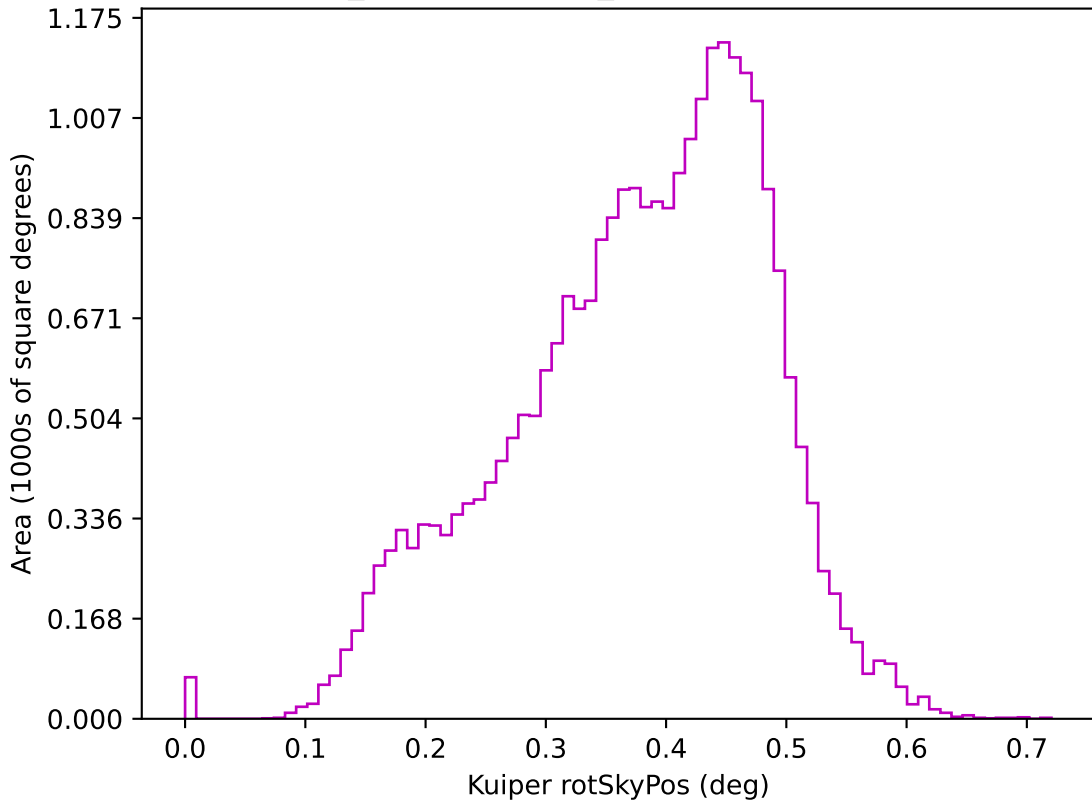
weather_cloudso36v3.5_10yrs z: Kuiper rotSkyPos
