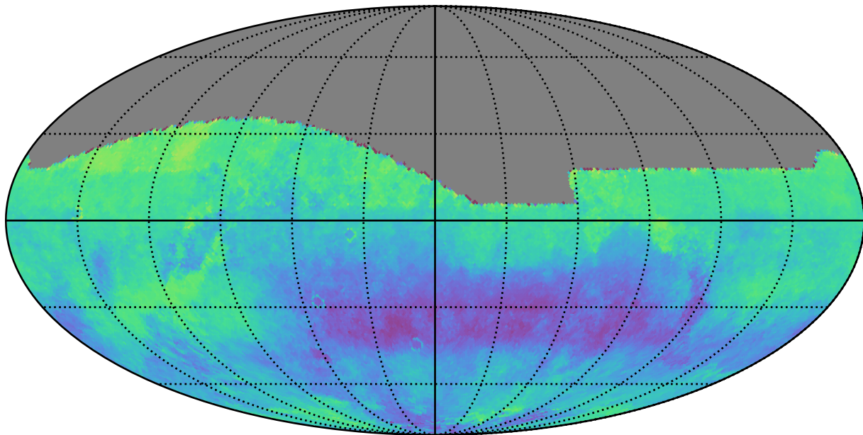
weather_cloudso36v3.5_10yrs z: Kuiper rotSkyPos
