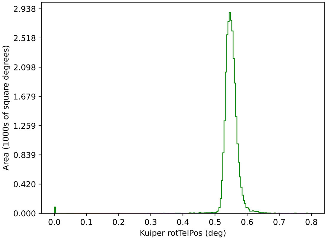
weather_cloudso36v3.5_10yrs g: Kuiper rotTelPos
