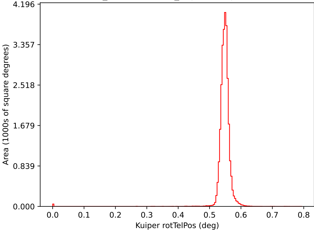
weather_cloudso36v3.5_10yrs i: Kuiper rotTelPos
