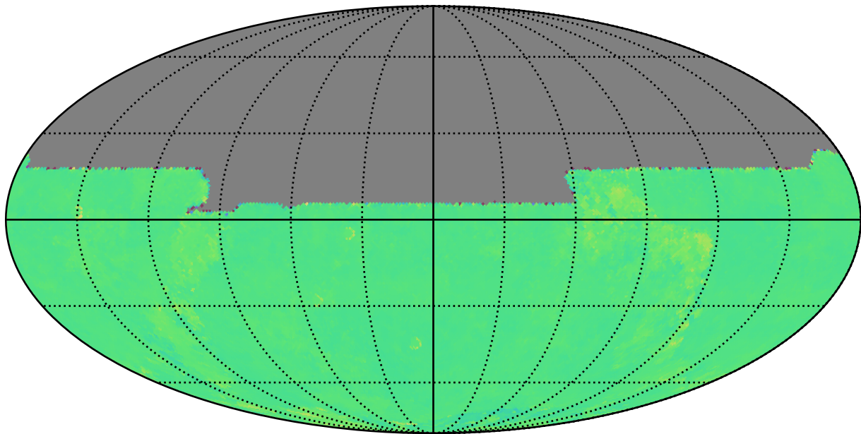
weather_cloudso36v3.5_10yrs y: Kuiper rotTelPos
