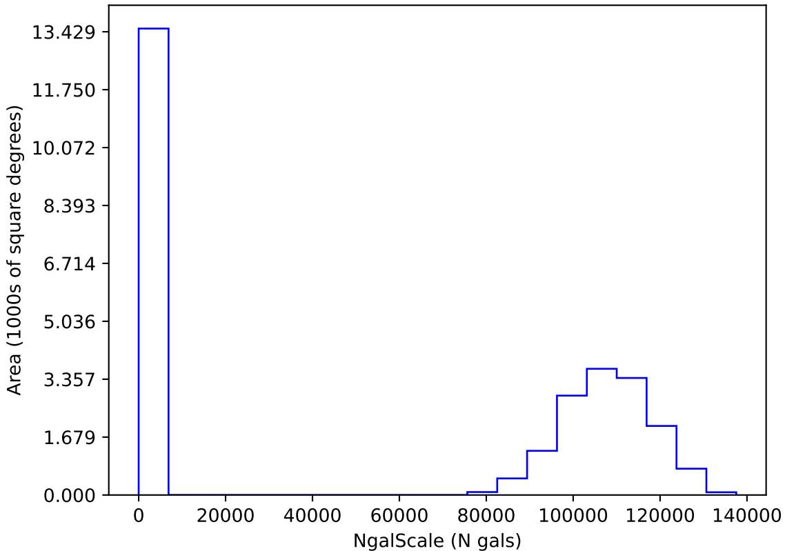
weather_cloudso36v3.5_10yrs i: NgalScale
