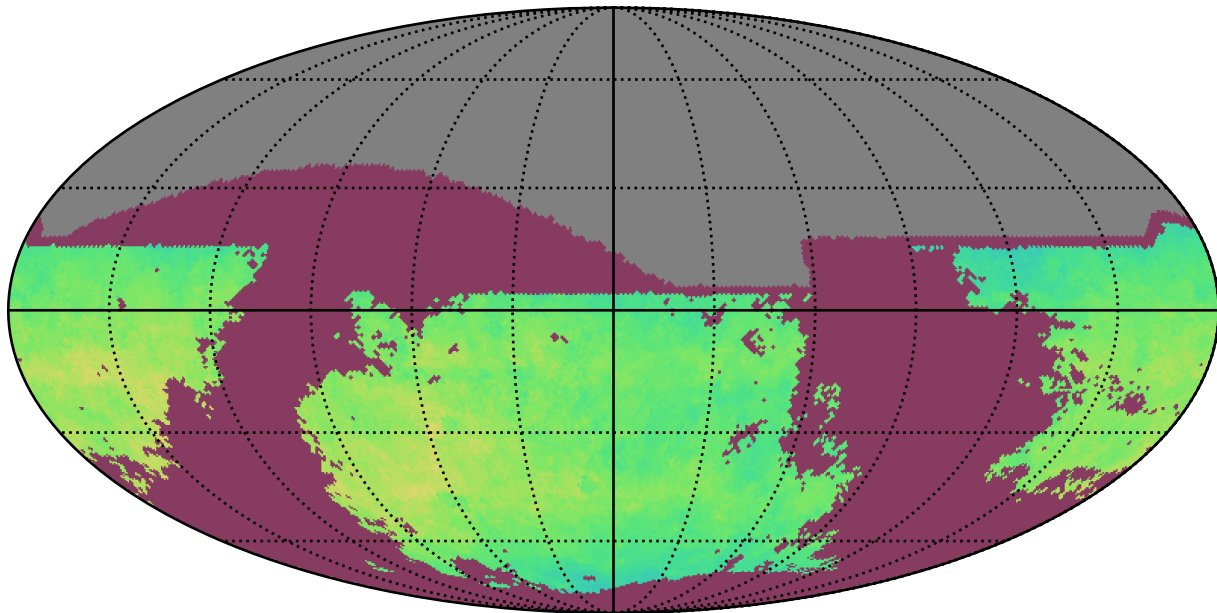
weather_cloudso36v3.5_10yrs i: NgalScale
