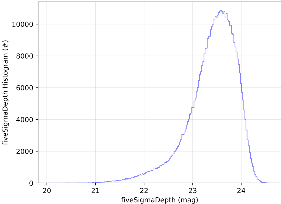
weather_cloudso36v3.5_10yrs i: fiveSigmaDepth Histogram
