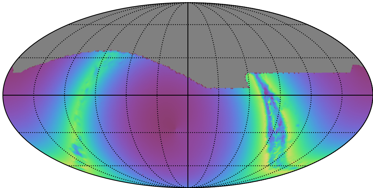
weather_cloudso36v3.5_10yrs : young_stars
