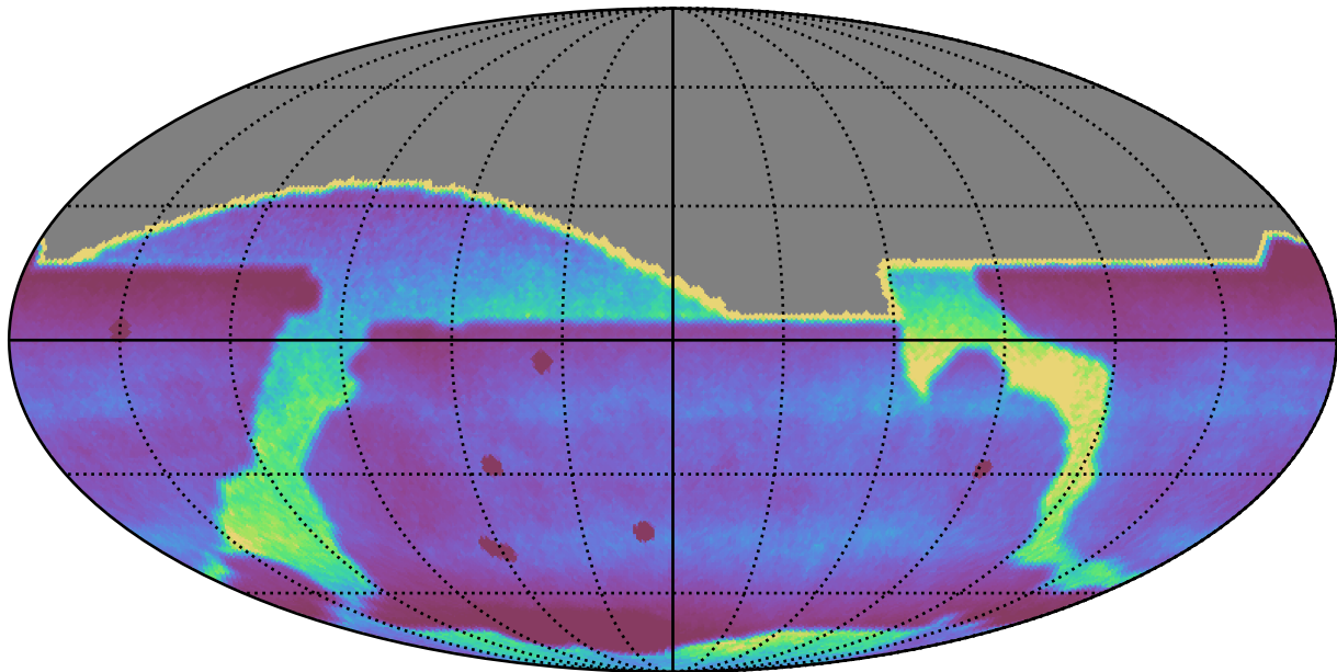
weather_cloudso4v3.5_10yrs : DCRprecision
