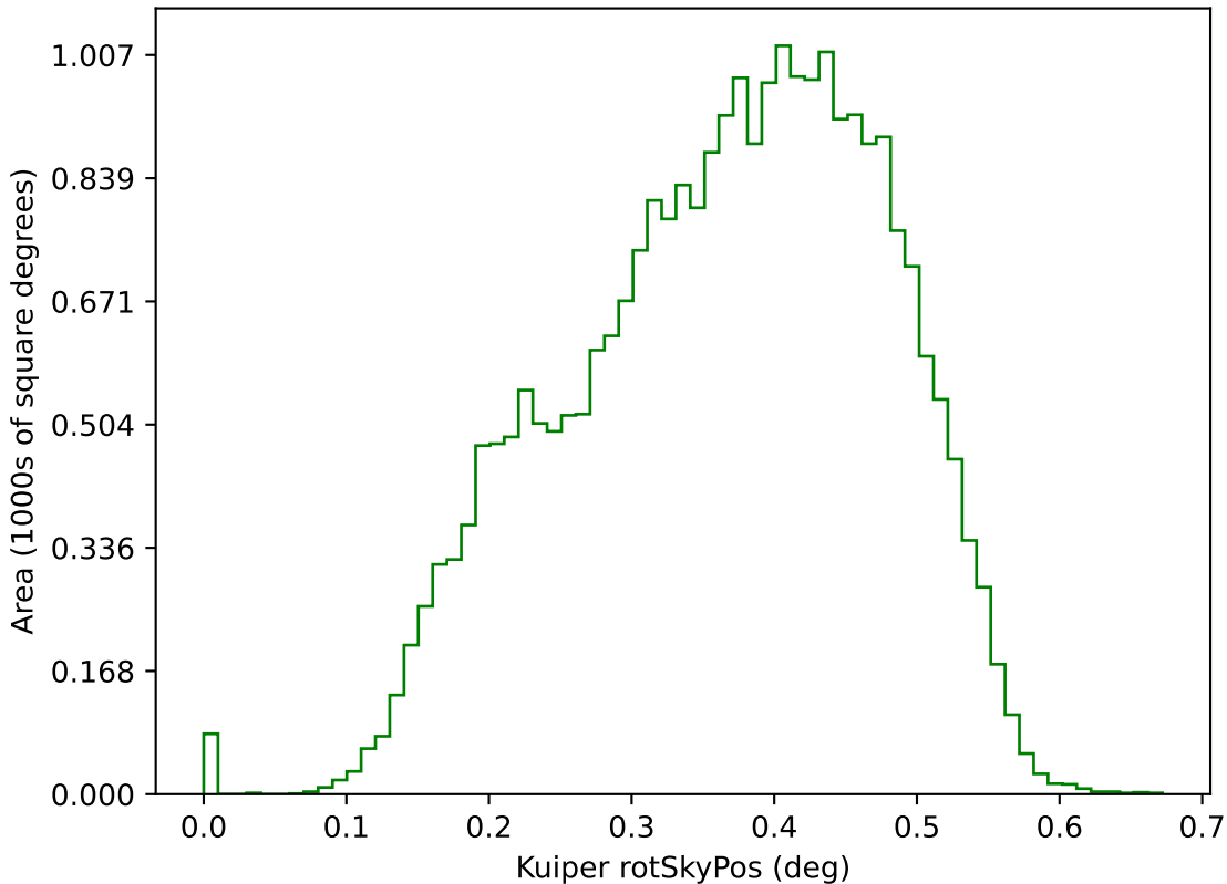
weather_cloudso4v3.5_10yrs g: Kuiper rotSkyPos
