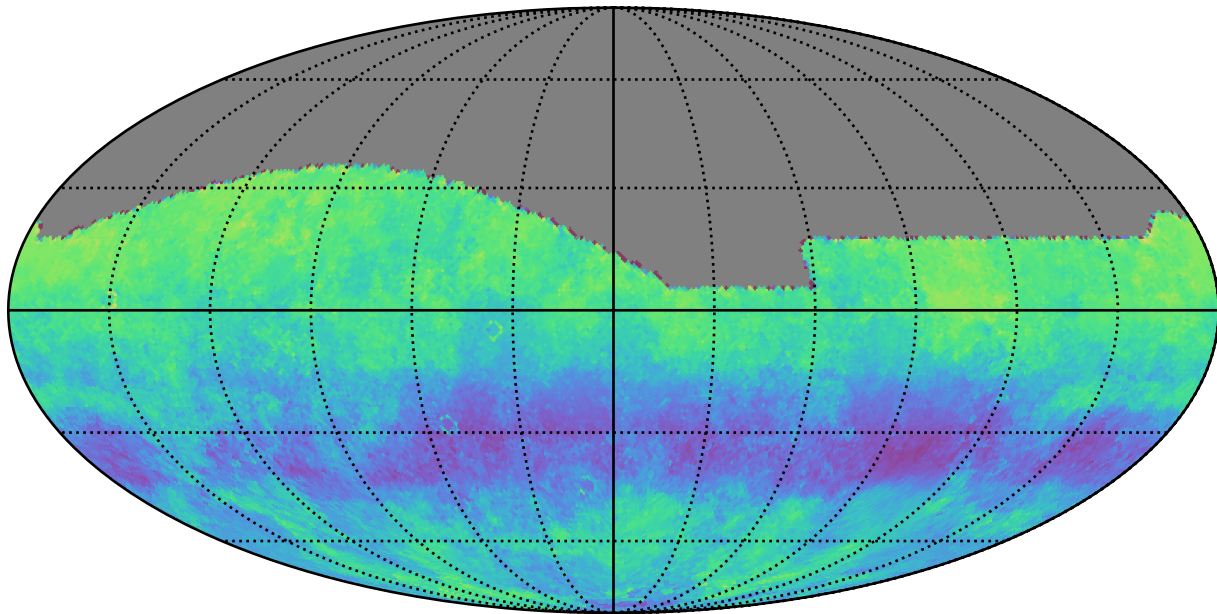
weather_cloudso4v3.5_10yrs g: Kuiper rotSkyPos
