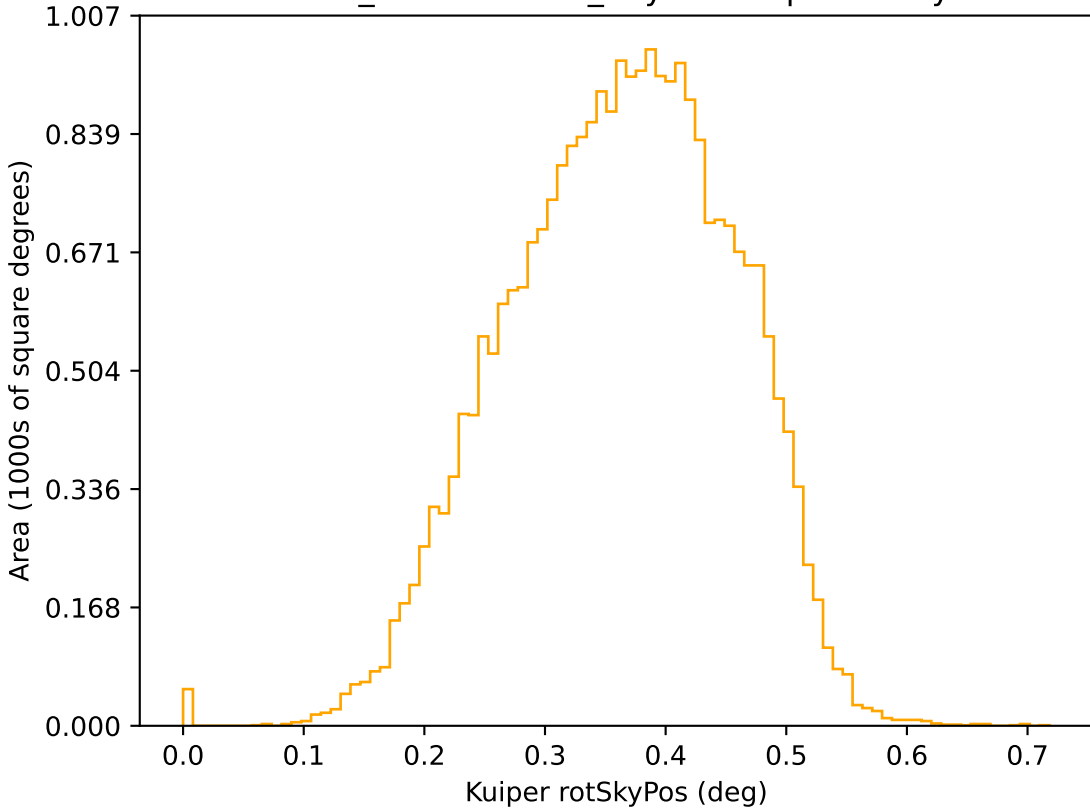
weather_cloudso4v3.5_10yrs r: Kuiper rotSkyPos
