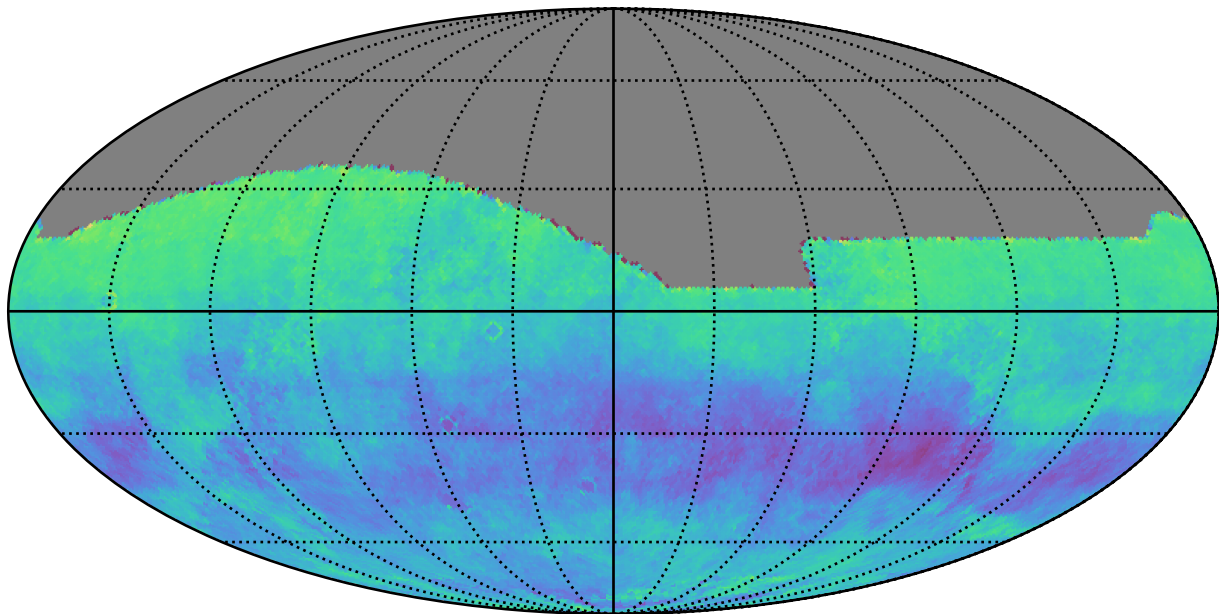
weather_cloudso4v3.5_10yrs r: Kuiper rotSkyPos
