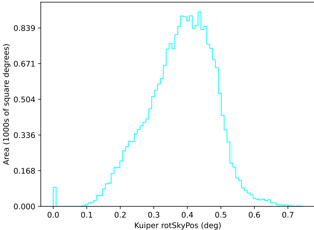
weather_cloudso4v3.5_10yrs u: Kuiper rotSkyPos
