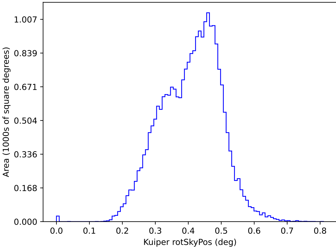
weather_cloudso4v3.5_10yrs y: Kuiper rotSkyPos
