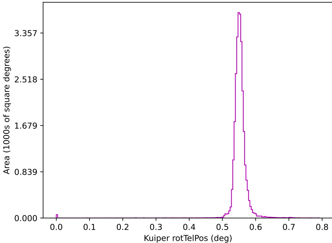
weather_cloudso4v3.5_10yrs z: Kuiper rotTelPos
