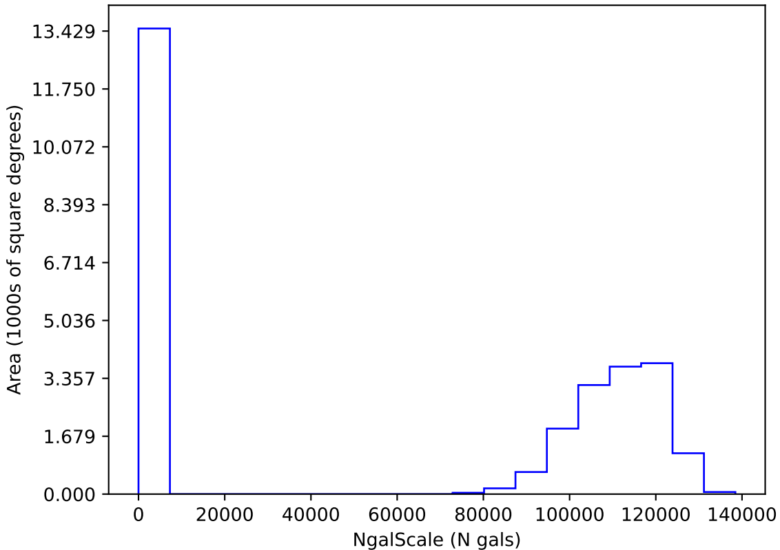
weather_cloudso4v3.5_10yrs i: NgalScale
