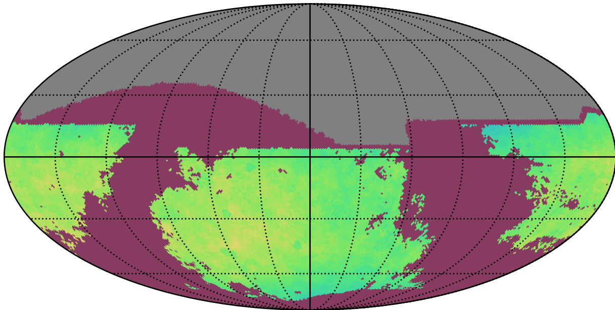
weather_cloudso4v3.5_10yrs i: NgalScale
