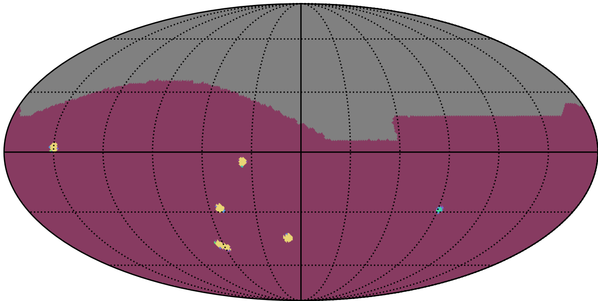
weather_cloudso4v3.5_10yrs : NumberOfQuickRevisits
