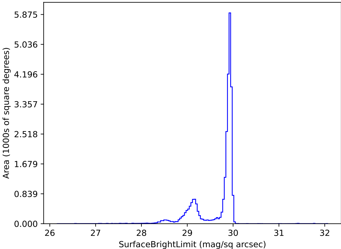
weather_cloudso4v3.5_10yrs i: SurfaceBrightLimit
