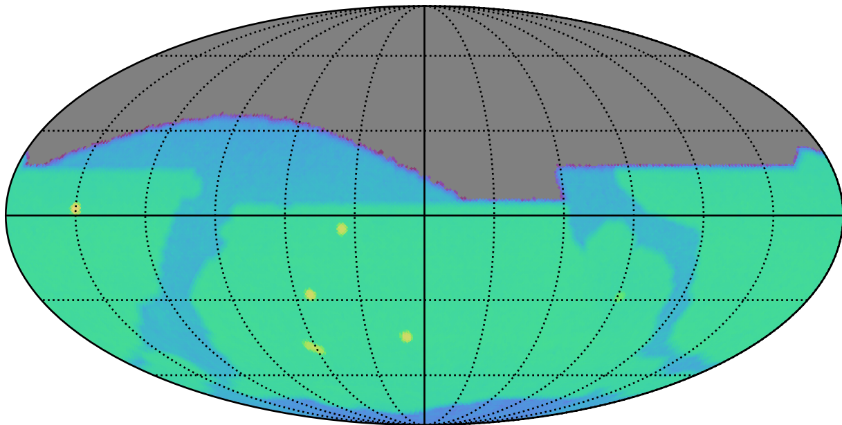
weather_cloudso4v3.5_10yrs i: SurfaceBrightLimit
