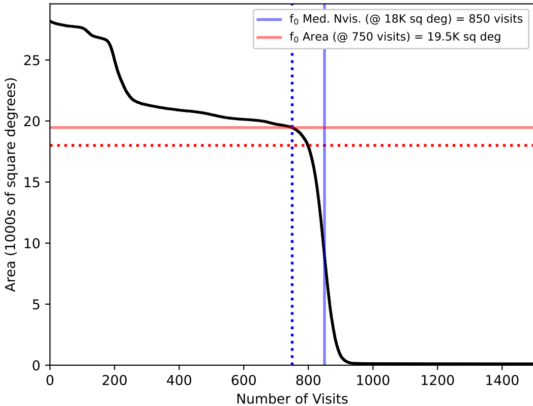
weather_cloudso4v3.5_10yrs : f0
