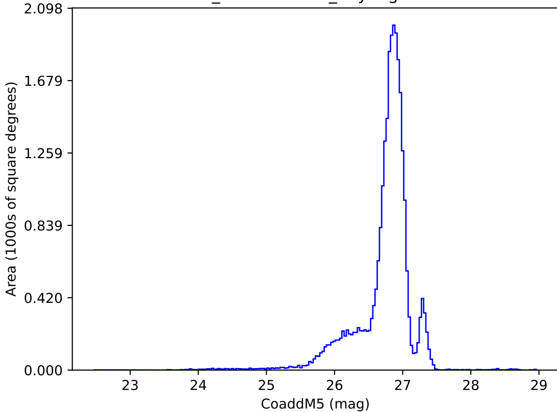
weather_cloudso6v3.5_10yrs g: CoaddM5
