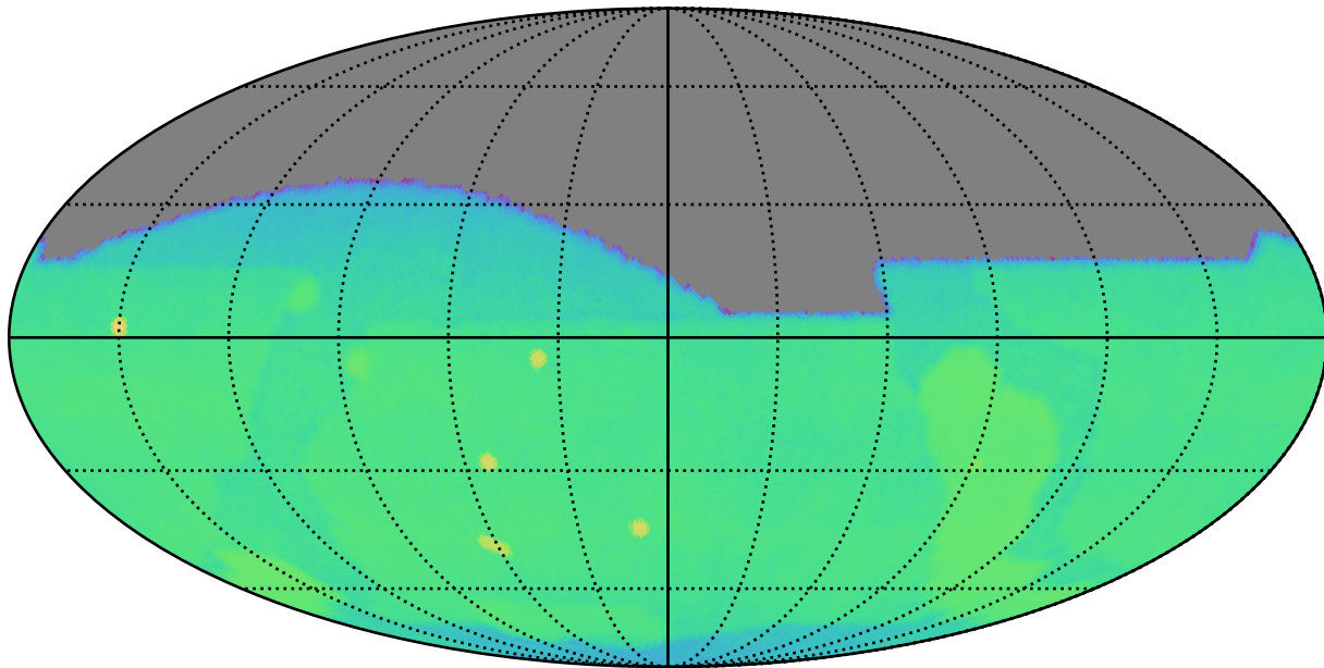
weather_cloudso6v3.5_10yrs g: CoaddM5
