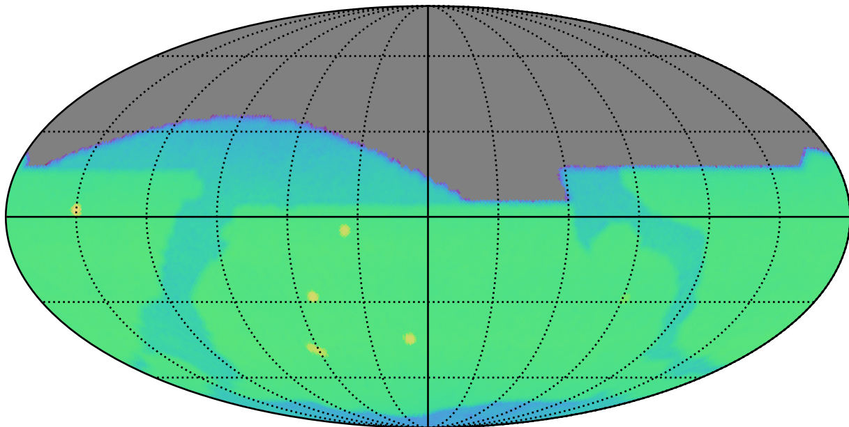
weather_cloudso6v3.5_10yrs i: CoaddM5
